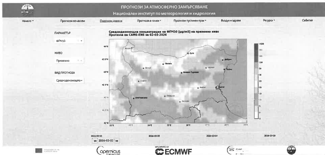
Фигура 4: Прогнози за атмосферно замърсяване от НИМХ
